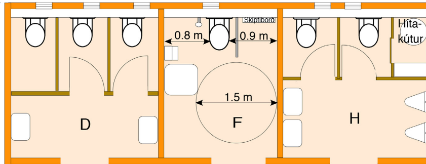
Grunnteikning af Contimade salernishúsi.
