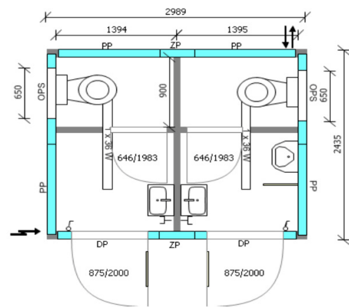
Grunnteikning af 10 feta Schafy salernishúsi.
